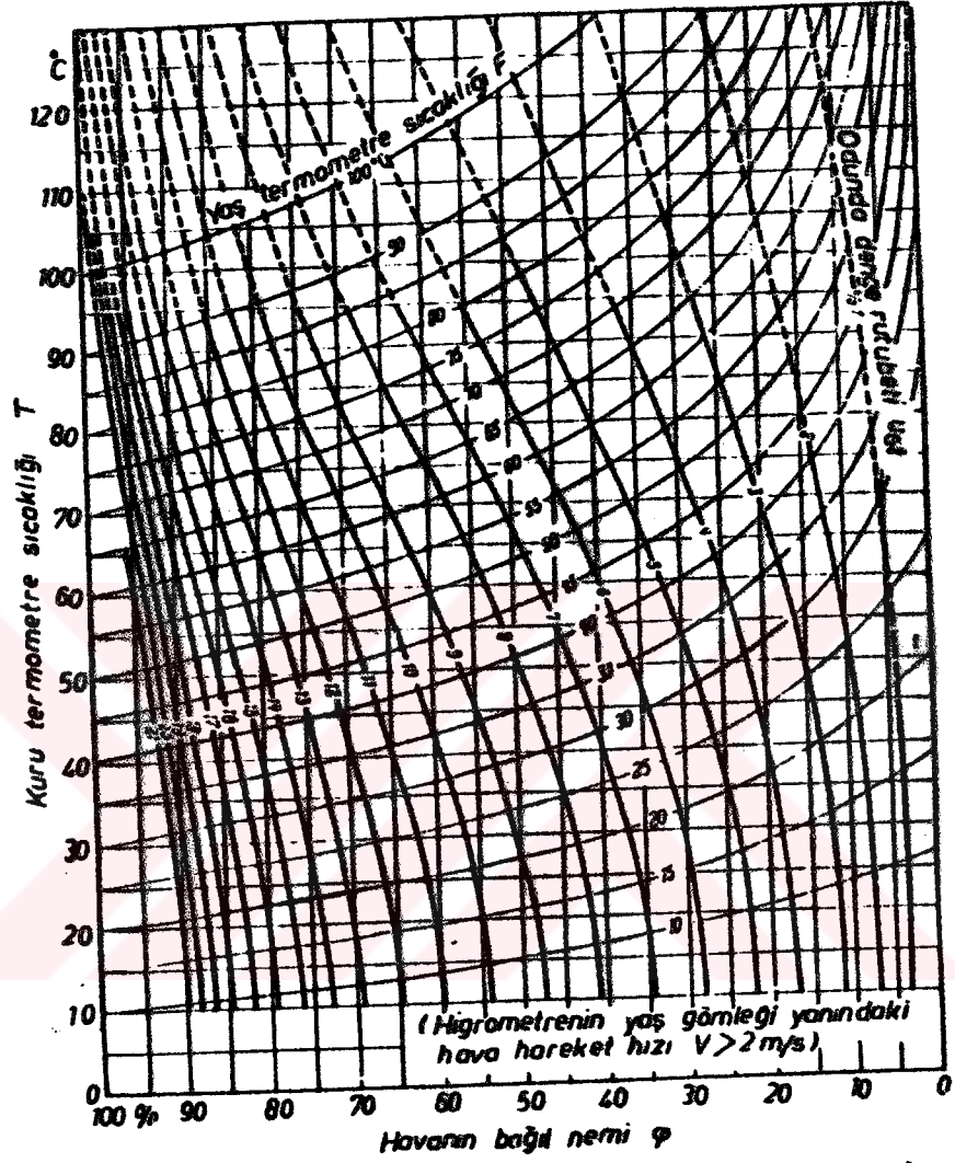
Şekil 4. Kuru termometre sıcaklığı, hava bağıl nemi, yaş termometre sıcaklığı ve denge rutubeti arasındaki ilişkiler (26).
