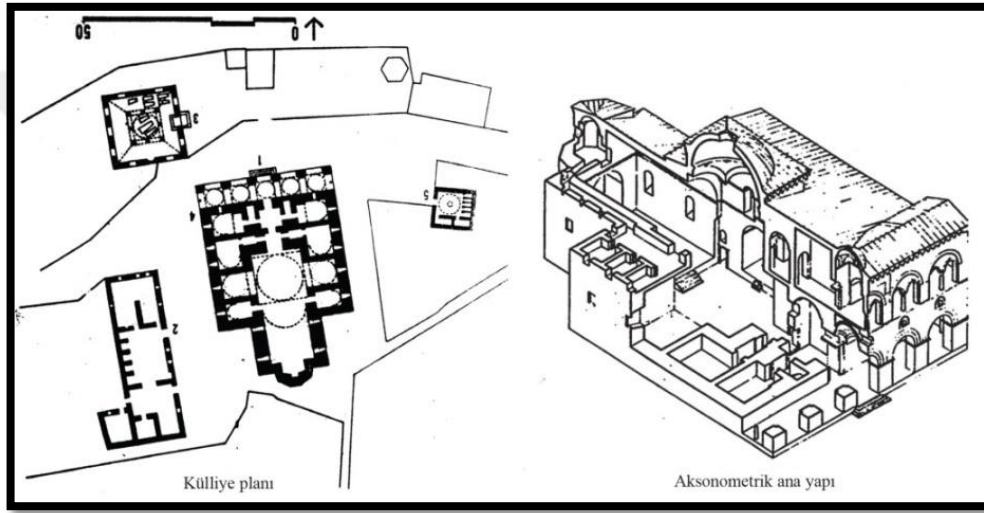
Şekil 3. Bursa Hüdavendigâr Külliyesi Vaziyet Planı, Cengiz Bektaş
