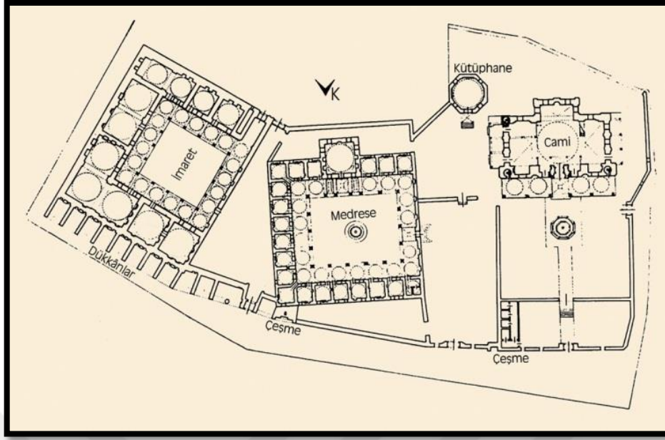
Şekil 75. Manisa Muradiye Külliyesi Vaziyet Planı, (Kaynak: URL-41)
