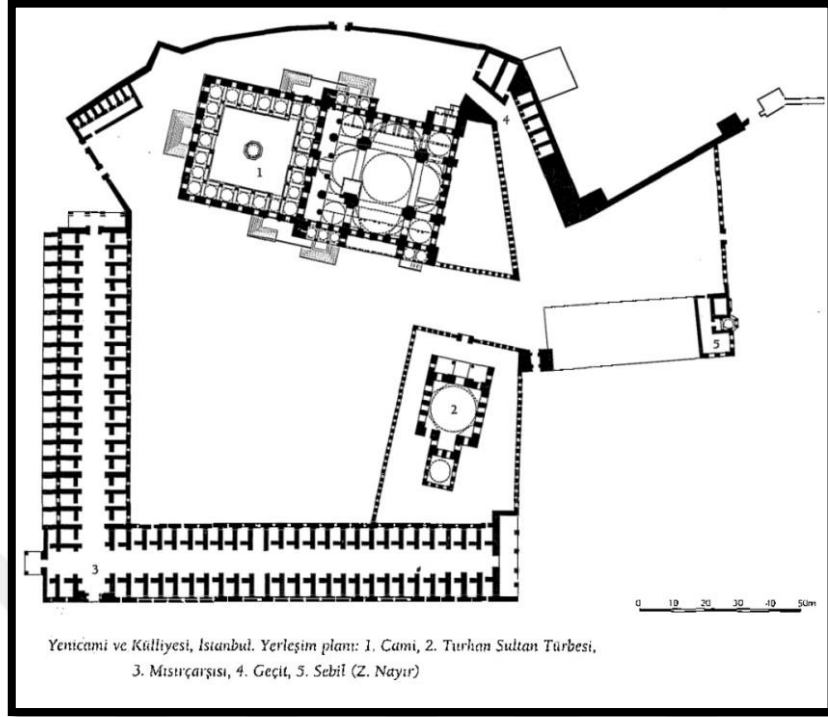
Şekil 84. Eminönü( İstanbul) Yeni Cami Külliyesi Vaziyet Planı, Z. Nayır
