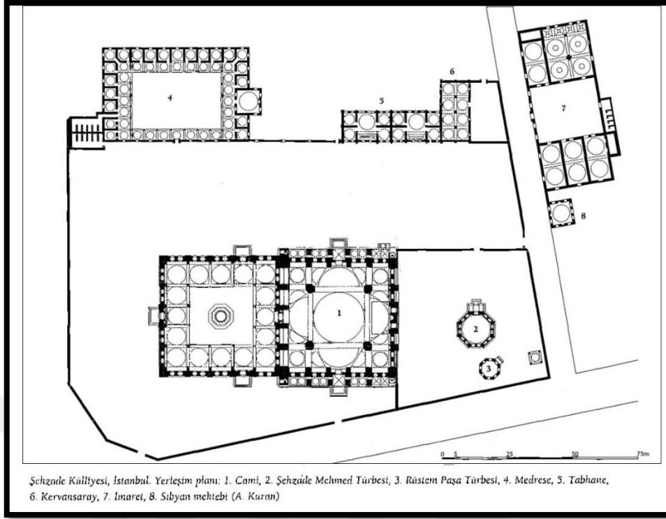
Şekil 59. İstanbul Şehzade Külliyesi Vaziyet Planı, A. Kuran
