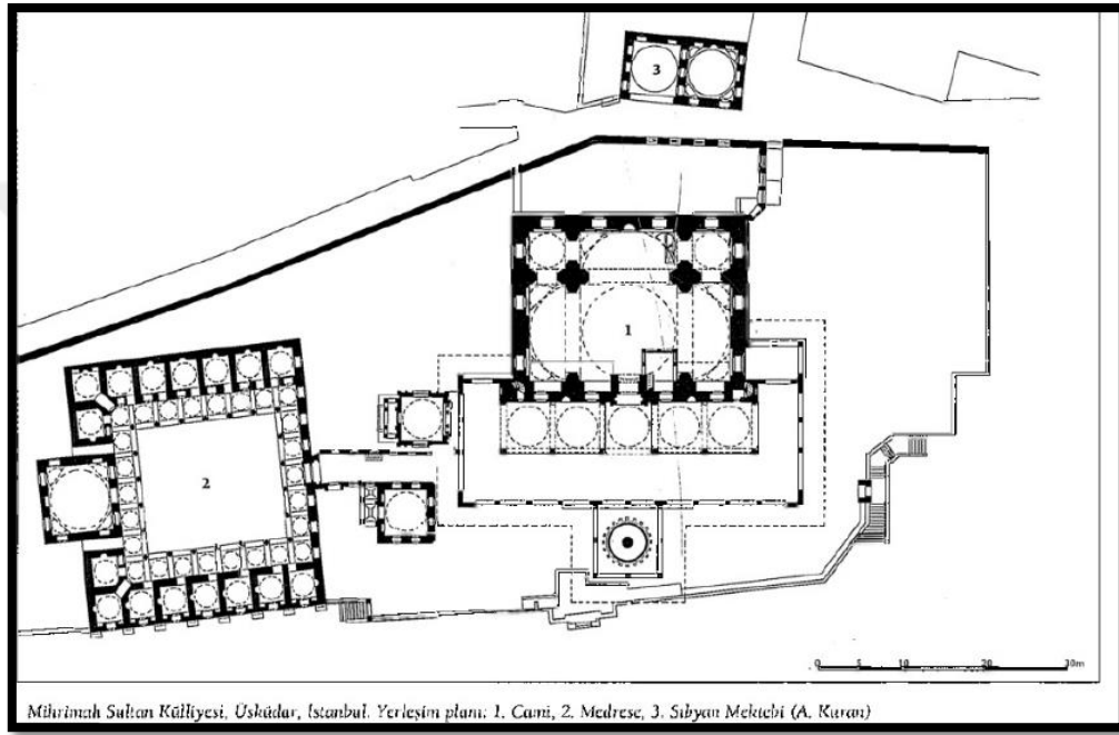
Şekil 56. Üsküdar (İstanbul) Mihrimah Sultan Külliyesi Vaziyet Planı, A. Kuran
