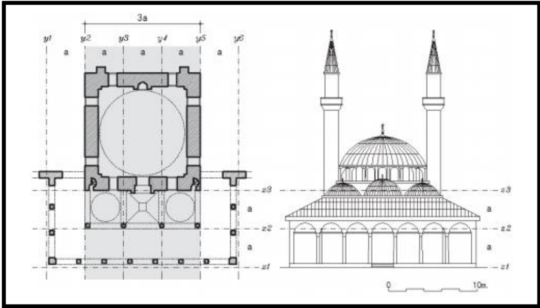
Şekil 62. Şam(Suriye) Süleymaniye Cami Plan ve Görünüşü, Nil Orbeyi
