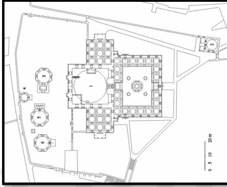
Şekil 54. İstanbul Yavuz Sultan Selim Külliyesi Vaziyet Planı,1-Cami, 2-Sıbyan Mektebi, 3-Yavuz Sultan Selim Türbesi, 4-Hafsa Sultan Türbesi, 5-Sultan Süleyman'ın Çocuklarının Türbesi, 6-Abdülmecid Türbesi, Müller-Wiener, Bildlexikon
