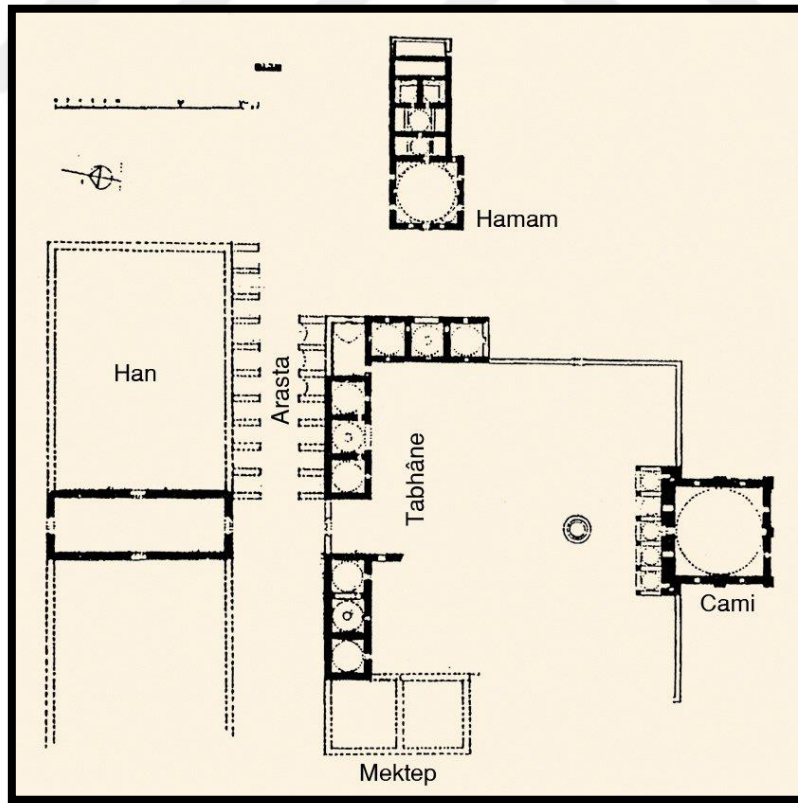
Şekil 66. Karapınar Sultan Selim Külliyesi Vaziyet Planı, (Kaynak:URL-38)
