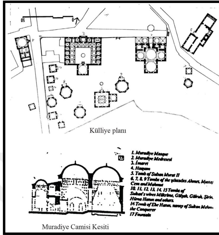
Şekil 24. Bursa Muradiye Cami ve Külliyesi Vaziyet Planı, Cengiz Bektaş
