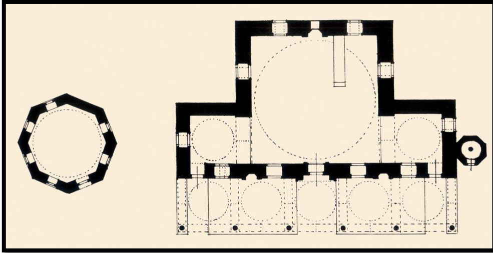
Şekil 51. Gülbahar Hatun Cami ve Türbesinin Planı, (Kaynak: URL-31)
