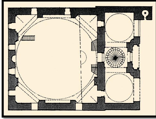
Şekil 10. Mudrunu Yıldırım Bayezid Cami Planı (Bolu), (Kaynak: URL-5)
