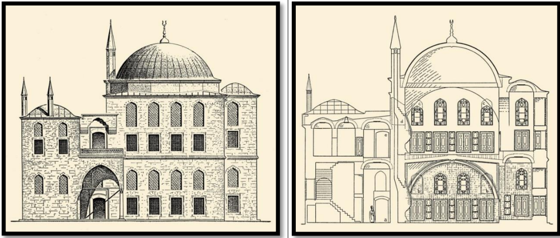
Şekil 82. İstanbul Davud Paşa Sarayı Güneybatı Görünüş ve Kesiti, Sedat Hakkı Eldem
