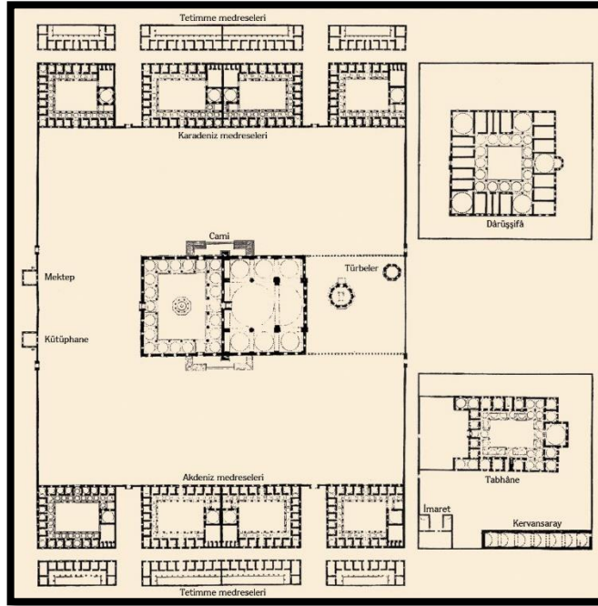
Şekil 38. İstanbul Fatih Cami ve Külliyesi Vaziyet Planı, (Kaynak: URL-25)
