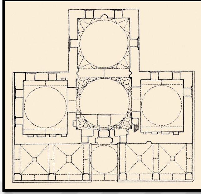
Şekil 26. Edirne Muradiye Cami Planı, (Kaynak: URL-17)
