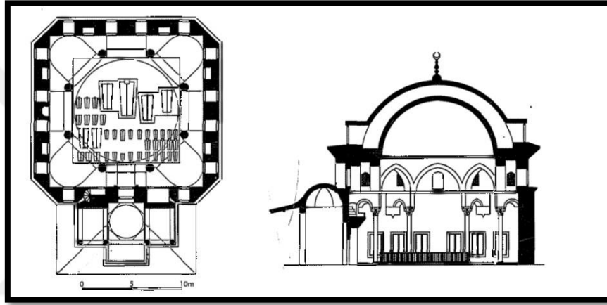
Şekil 71. İstanbul II. Selim Türbesi Plan ve Kesiti , A. Kuran
