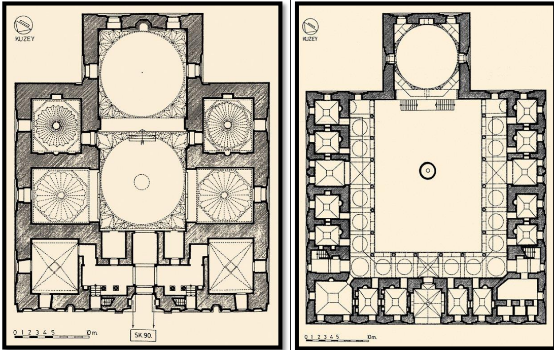
Şekil 20. Bursa Yeşil Cami ve Medresesi Planı, (Kaynak: URL-13)
