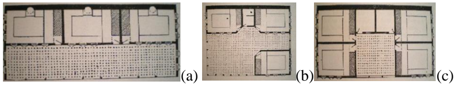
Şekil 12. a. Dış Sofalı Sıra Odalı Plan Tipi b. Dış Sofalı Köşk Odalı Plan Tipi c. Dış Sofalı Eyvanlı Plan Tipi (Eldem, 1986, 34).
