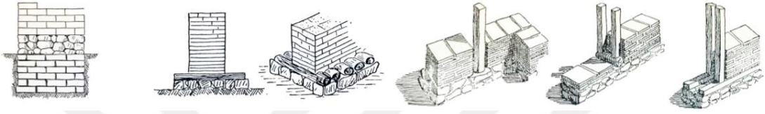
Şekil 16. Geleneksel konutlardaki duvar yapım teknikleri (Nauman, 1975,62-110)
