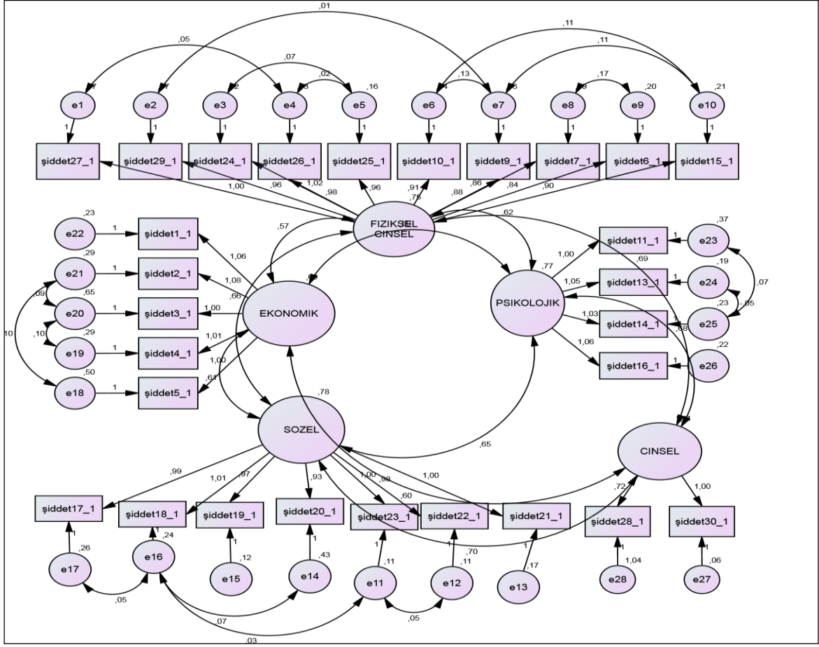
Şekil 3: Kadınların Şiddet Algısı Ölçeği DFA Sonuçları
